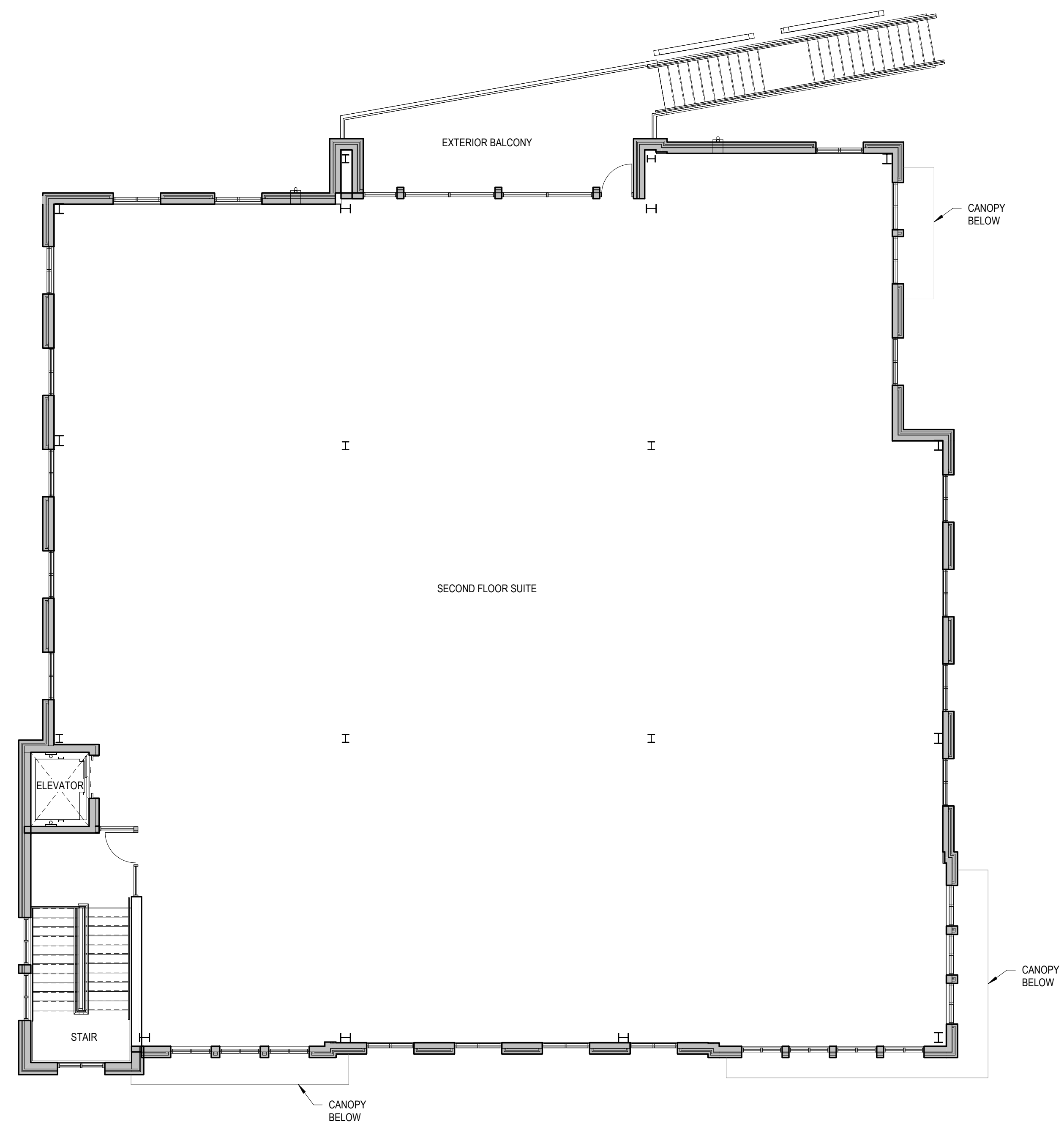
1 Level 2 - Floor Plan SK-3 SCALE: 1/8" = 1'-0"
